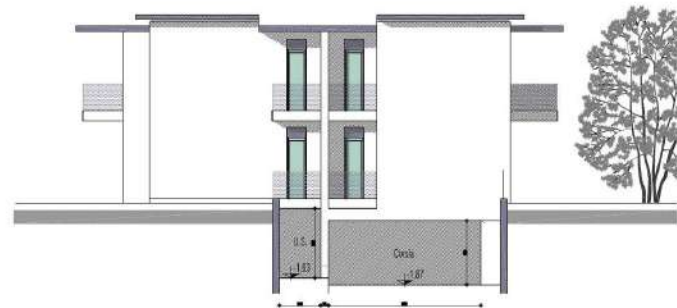
PROSPETTO NORD
